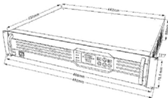
1-3 KVA Inverter
