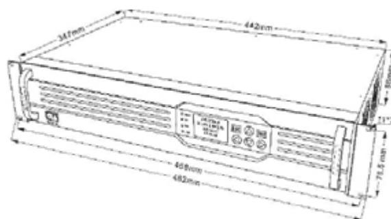
4-6 KVA Inverter
