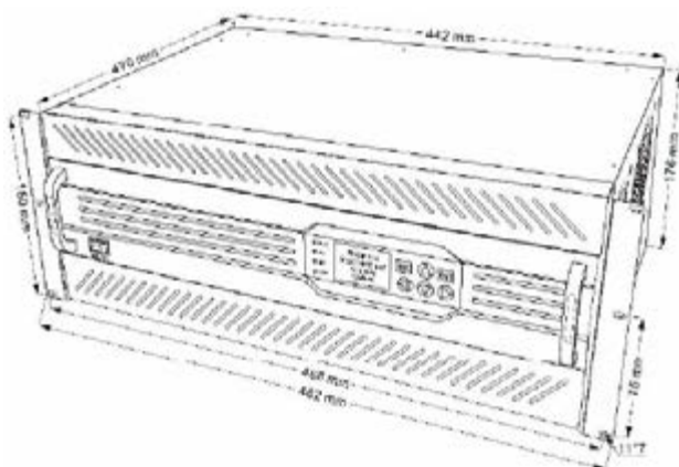
8-10 KVA Inverter
